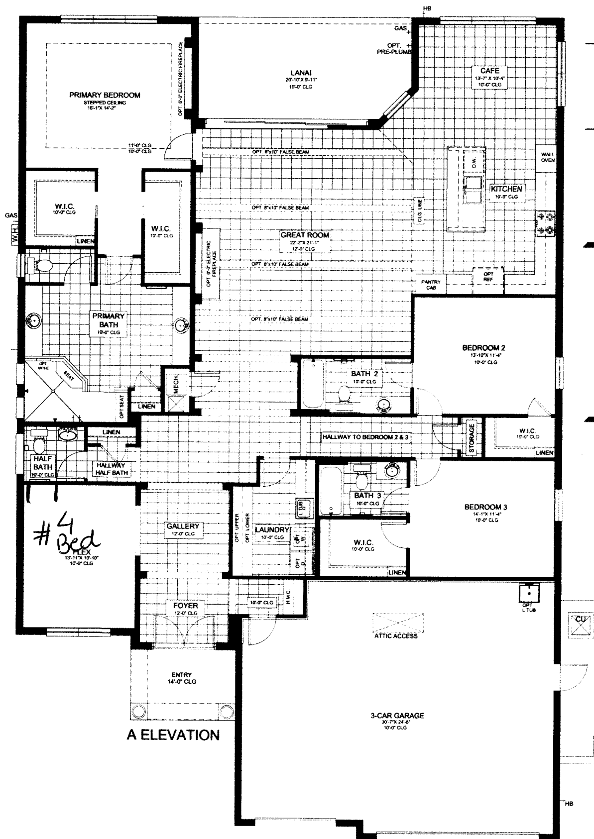
ELEVATION A
